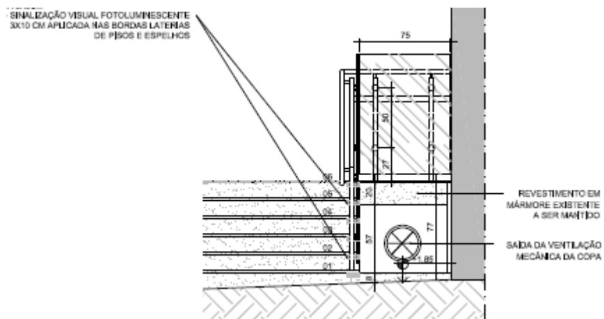
Vista guarda-corpo e corrimão da escada de acesso externo
