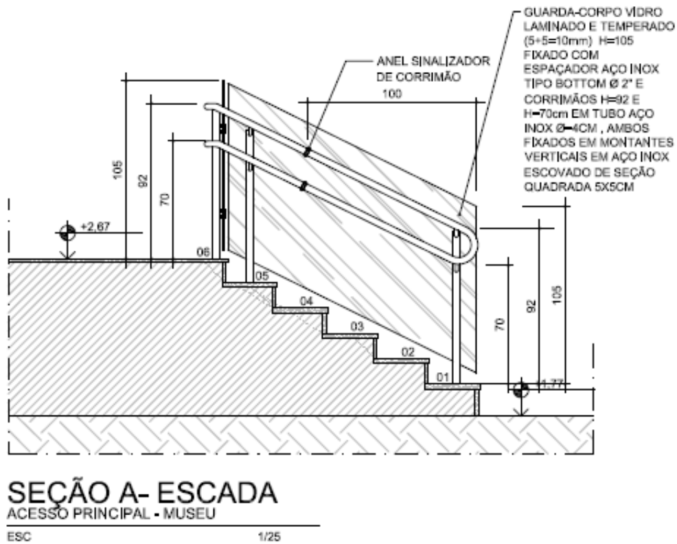
Seção guarda-corpo e corrimão da escada de acesso externo
