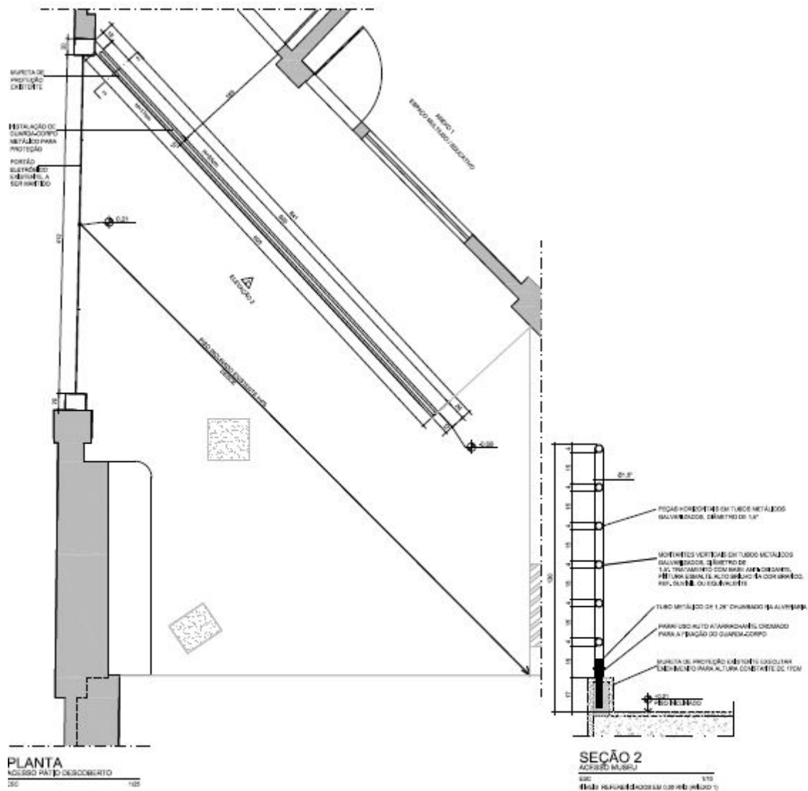
Planta e seção do Guarda corpo da entrada de veículos
