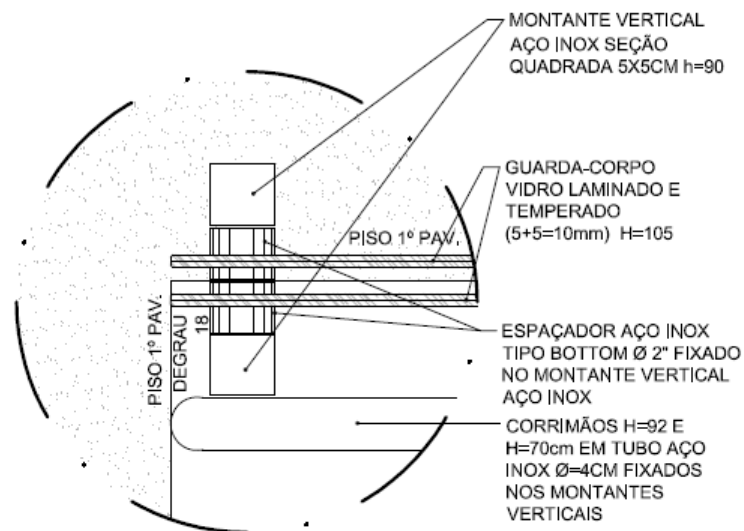
DETALHE 2 GUARDA-CORPO E CORRIMÃO AÇO INOX ESC 1/5
