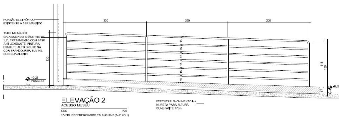
Elevação do Guarda corpo da entrada de veículos
