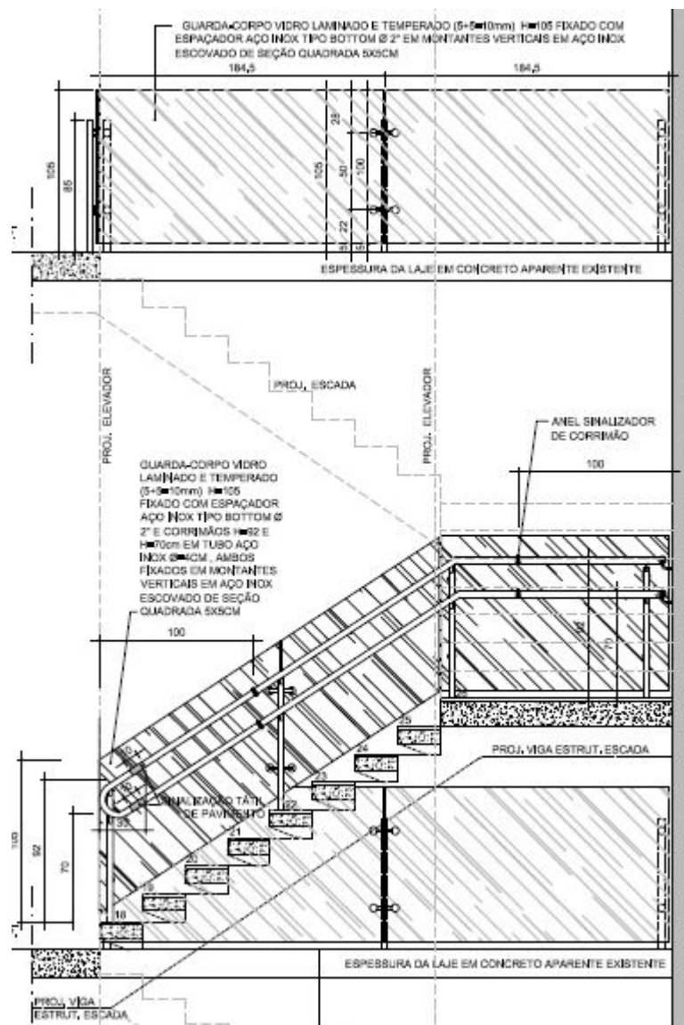
Seção escada interna com vista do guarda corpo e corrimão
