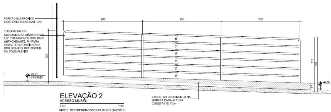
Elevação do Guarda corpo da entrada de veículos
